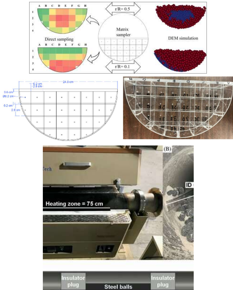
Figures 1–3 : Fours rotatifs et outil d'échantillonnage
